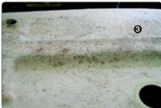
Problemzonen bei herkömmlichen Systemen: Hohlraum zwischen Träger und Wanne
